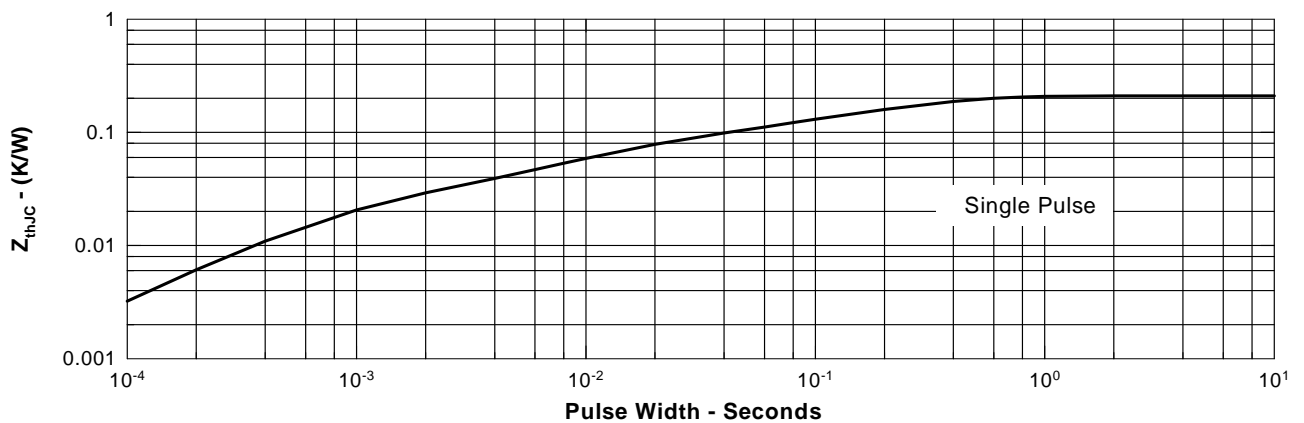
Fig. 10. Thermal Impedance
