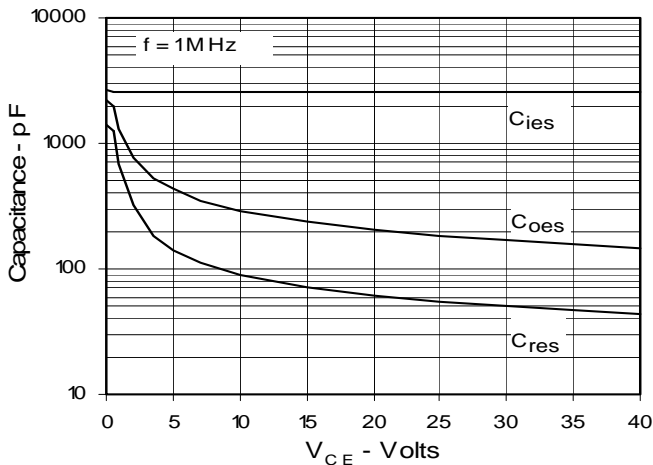
Fig. 12. Capacitance
